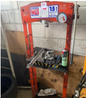
Sealy 15 ton YK15M press
